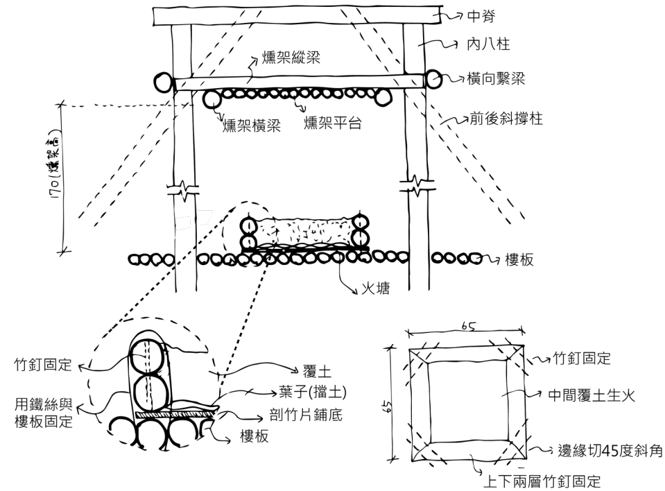
火塘平面圖
