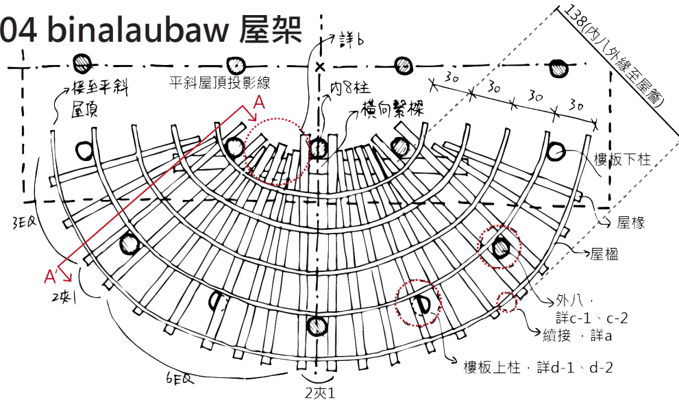
binalaubaw平面圖
