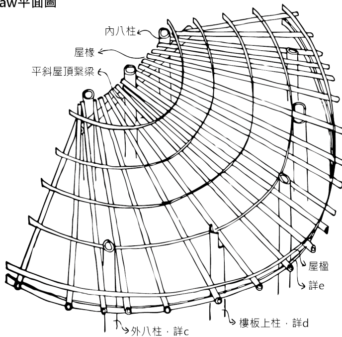
binalaubaw透視圖
