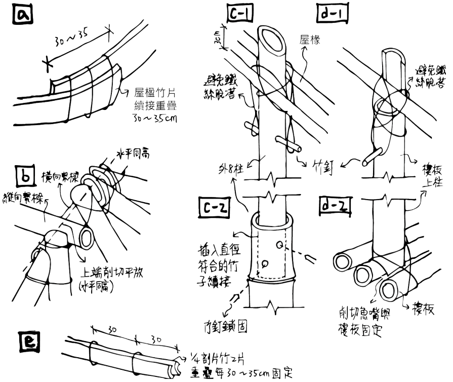
binalaubaw細部
