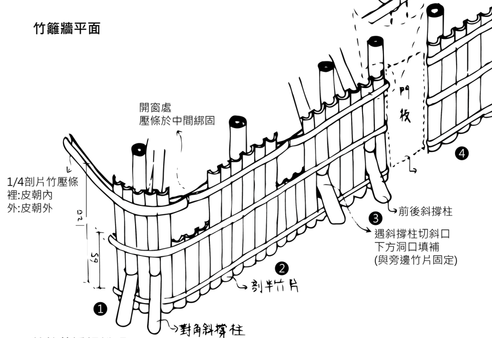
竹籬牆透視說明
