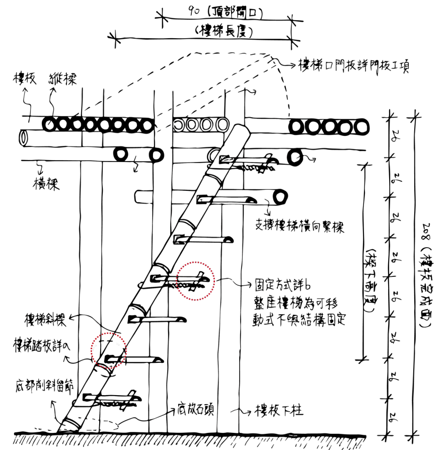
樓梯剖透
