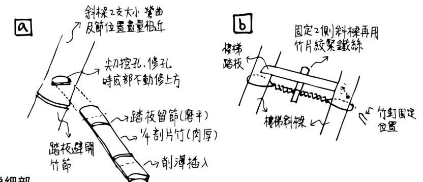
樓梯細部
